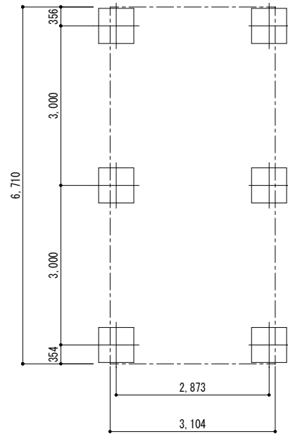
■ 基礎配置図
