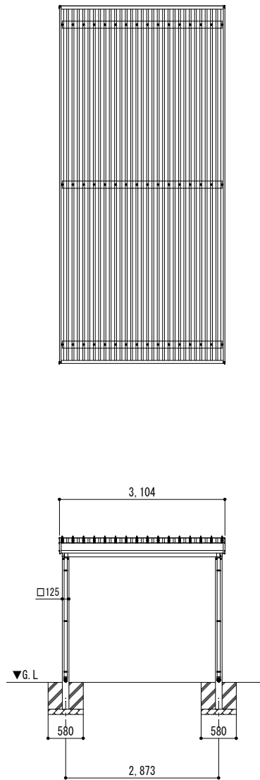
■ 断面図
